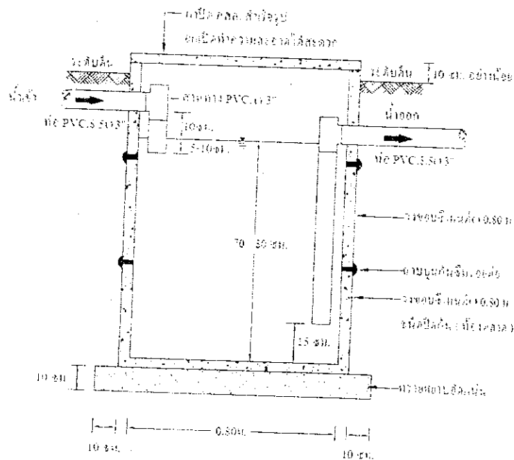
ข) แปลนภาพตัดขวางตามแนว A-A บ่อตกไขมันแบบวงขอบซีเมนต์
