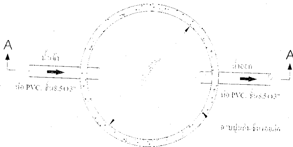
ก) แปลนภาพด้านบนของบ่อตัดไชนันแบบวงขอบซีเมนต์
